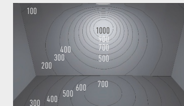
標:W900、H450、D300mm 取付位置:前から130mm
