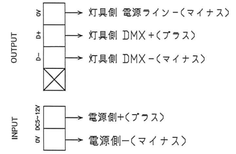
A部詳細
