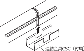
(図1) 連結金具CSCの取付方法 器具を突き合わせてコネクタを器具内へ収納してください。
