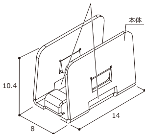
モジュールホルダー取付穴
