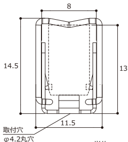
モジュールホルダー取付時
