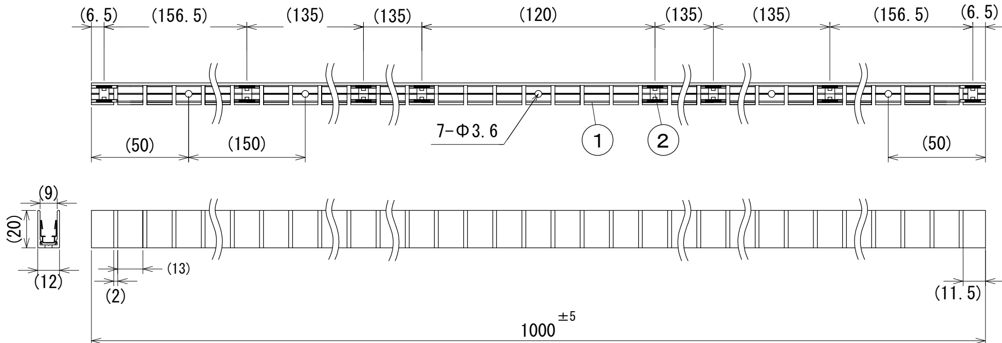
■LEDモジュール取付図 (1/1)
