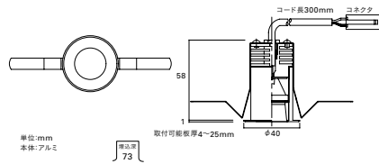
寸法図 コンパクトダウンライト DX233
