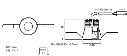
寸法図 ベースダウンライト DX203
