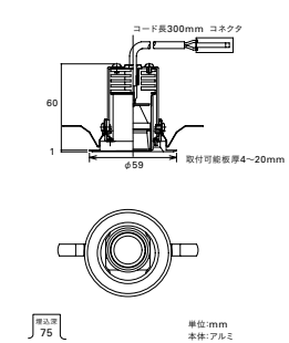
寸法図 ユニバーサルダウンライト DX223
