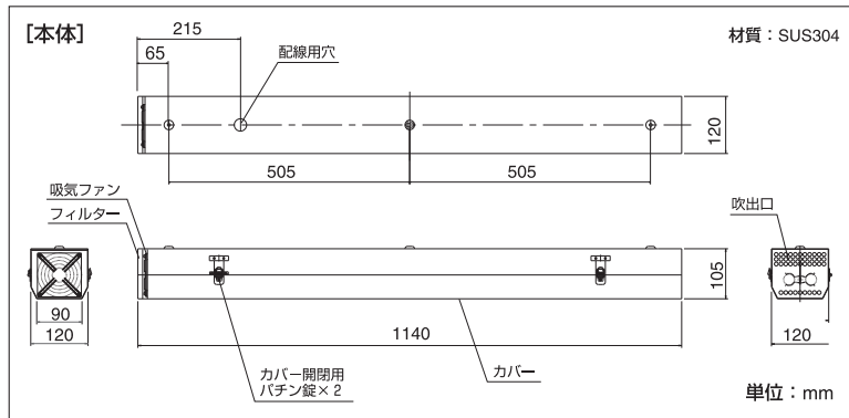
外形寸法
