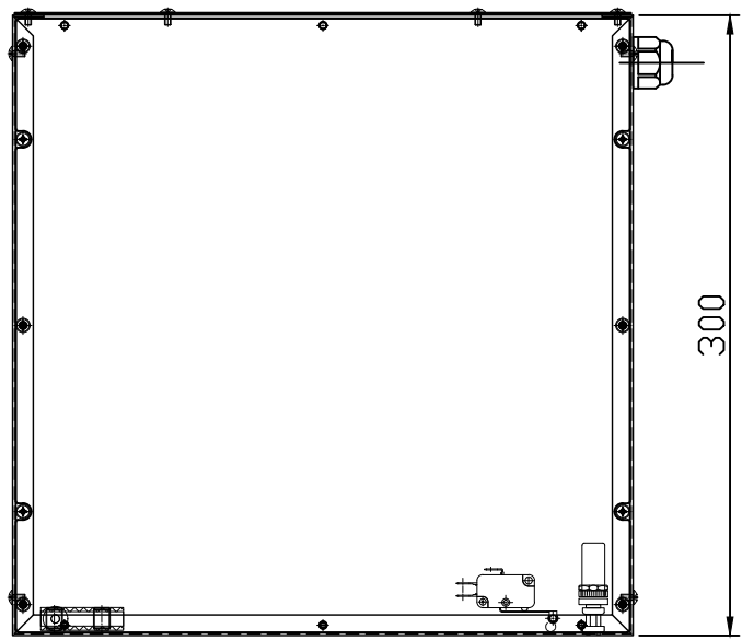
納入仕様図面
