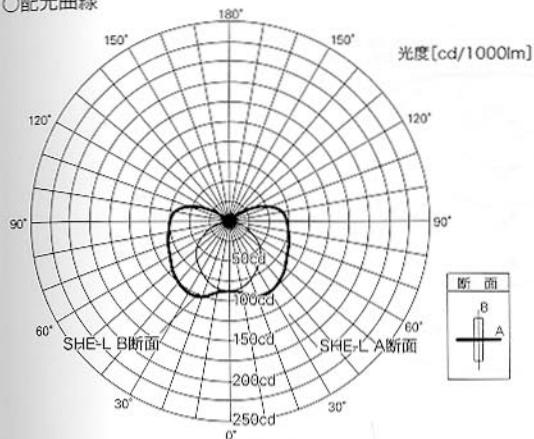
○配光曲線
