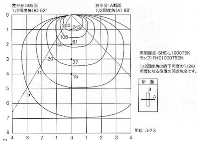
○水平面照度曲線
