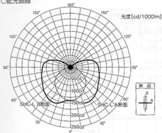
○配光曲線
