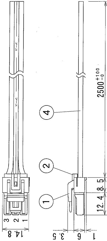
〔コネクタ正面図〕
