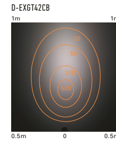
灯具高さ275mm 照射角度50° (単位:lx 写真は4000K)
