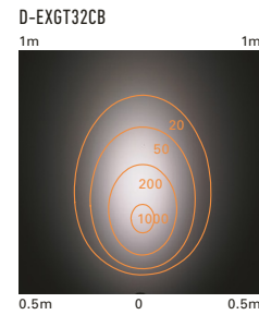
灯具高さ200mm 照射角度50° (単位:lx 写真は4000K)
