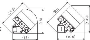
LEDモジュール取付時の寸法
