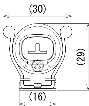
【20LYVホルダー（別売）取付図】
