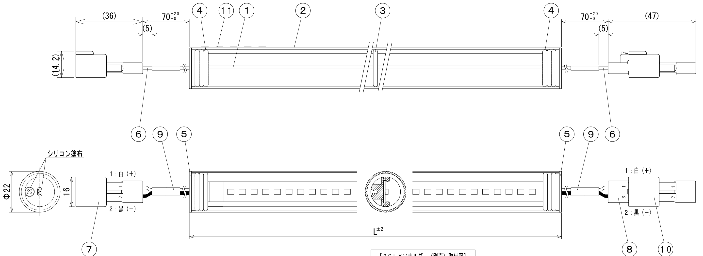
【20LYVホルダー（別売）取付図】
