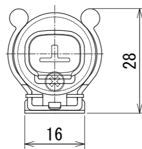
【20LYVホルダー（別売）取付図】
