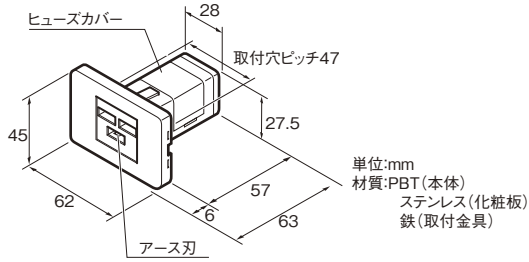
○埋込寸法と接続電線
