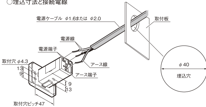
○埋込寸法と接続電線
