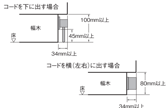
○コネクタおよびコードの収まり寸法
