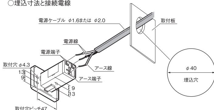
○埋込寸法と接続電線
