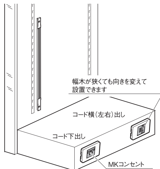
○コネクタおよびコードの収まり寸法
