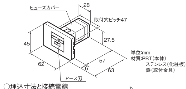
○埋込寸法と接続電線
