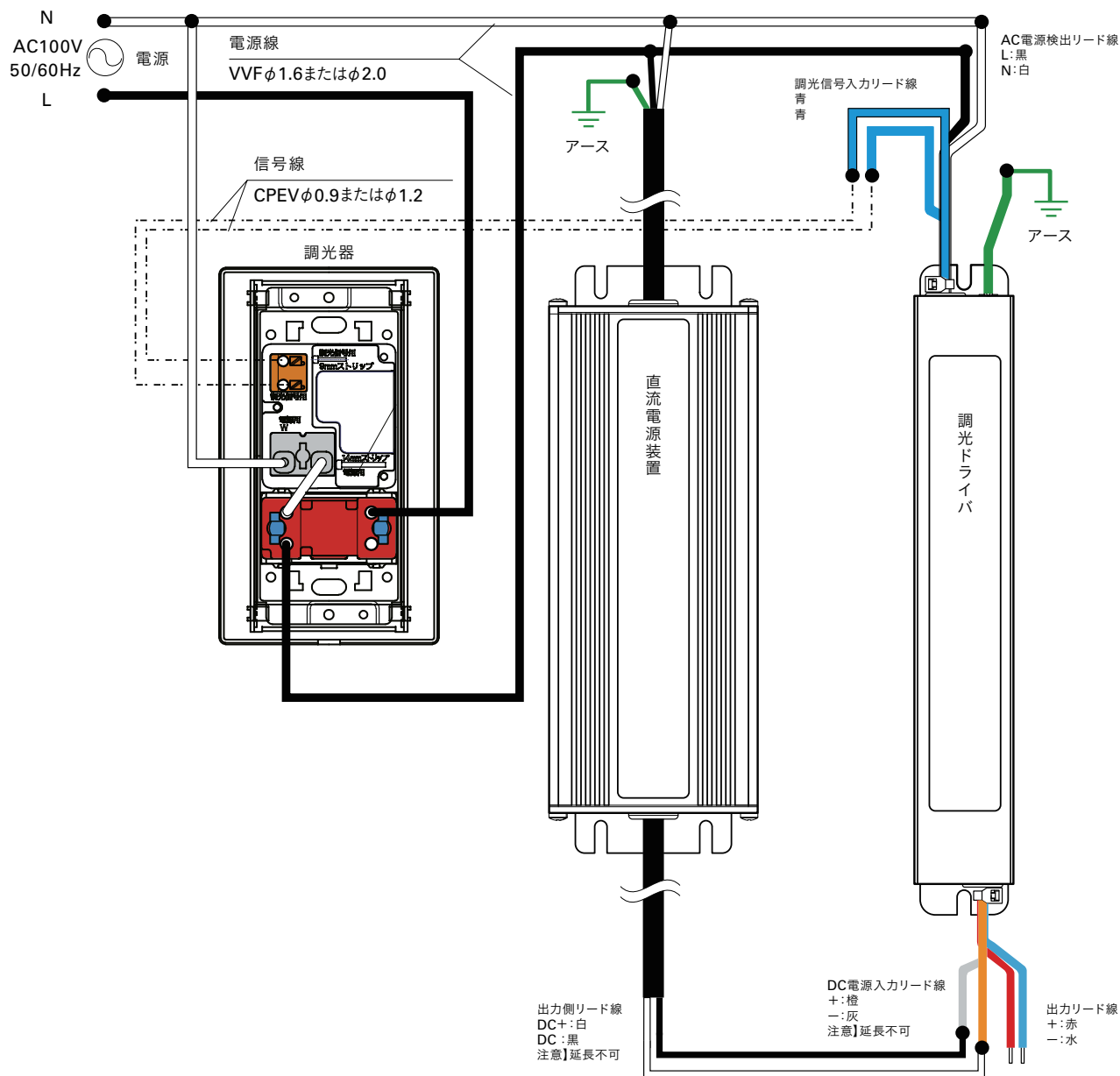
直流電源装置 ELD2475F + PWM調光ドライバ(調光下限1%) PDD240D
