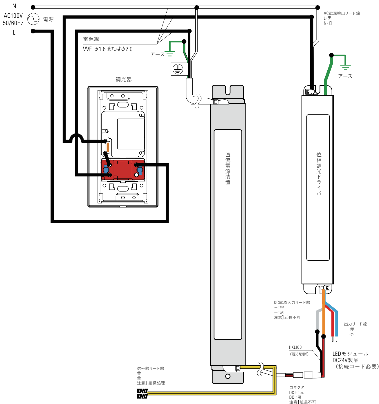
直流電源装置 ELD2-2435FD+位相調光ドライバ PDD240DB
