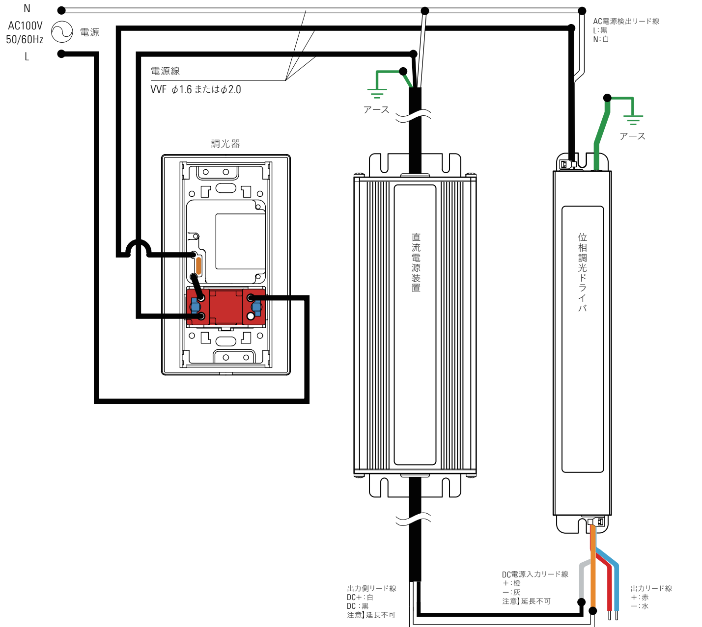
直流電源装置 ELD2475F+位相調光ドライバ PDD240DB
